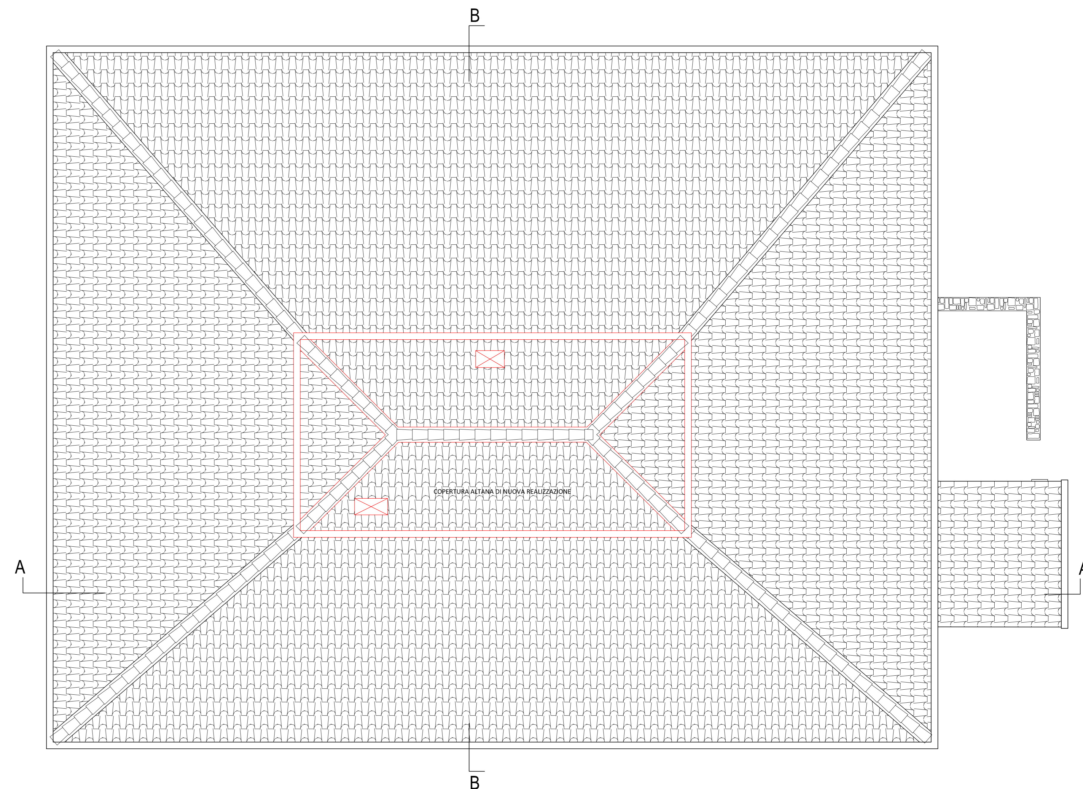
PIANTA COPERTURA
