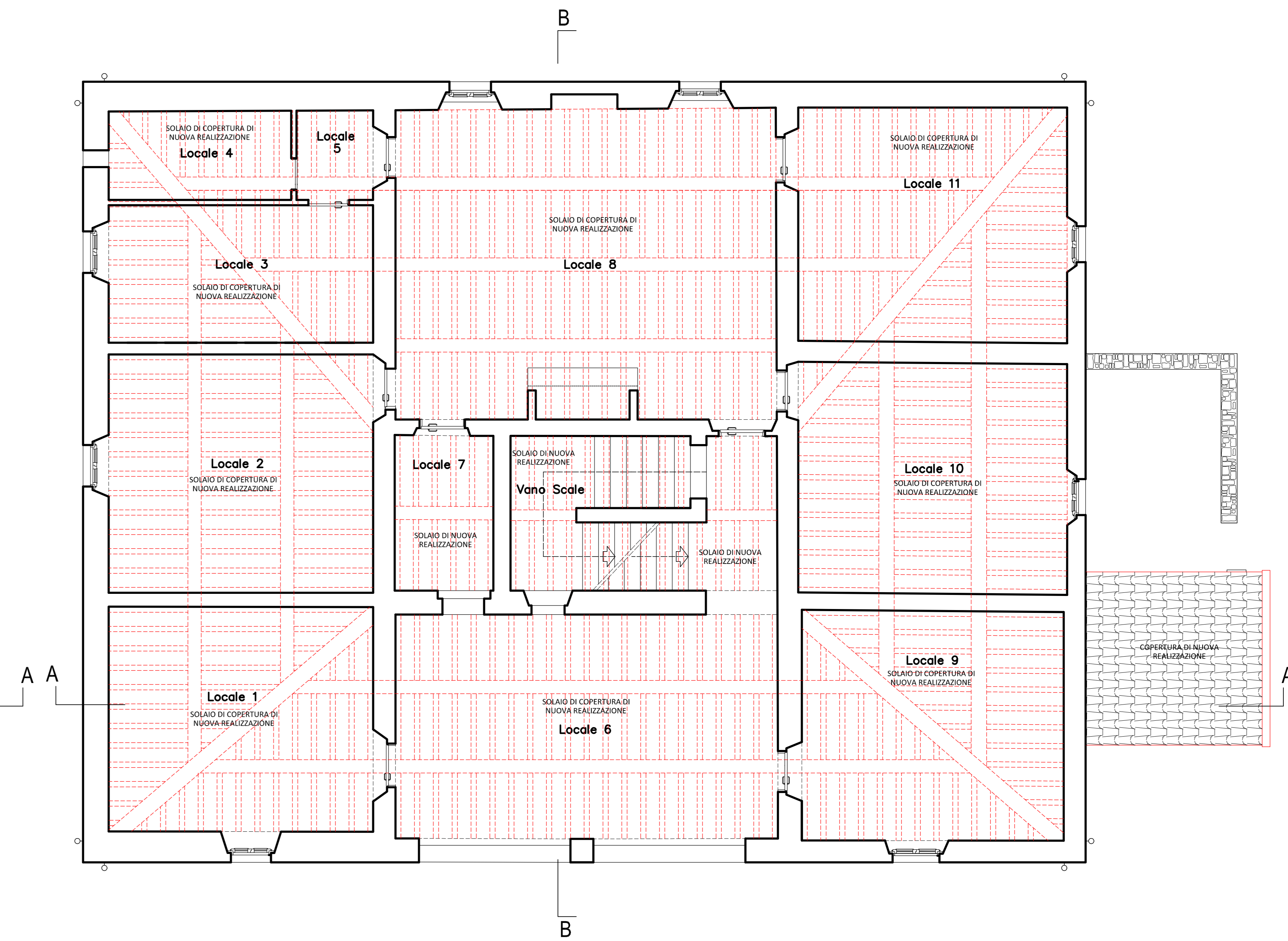
PIANO PRIMO
