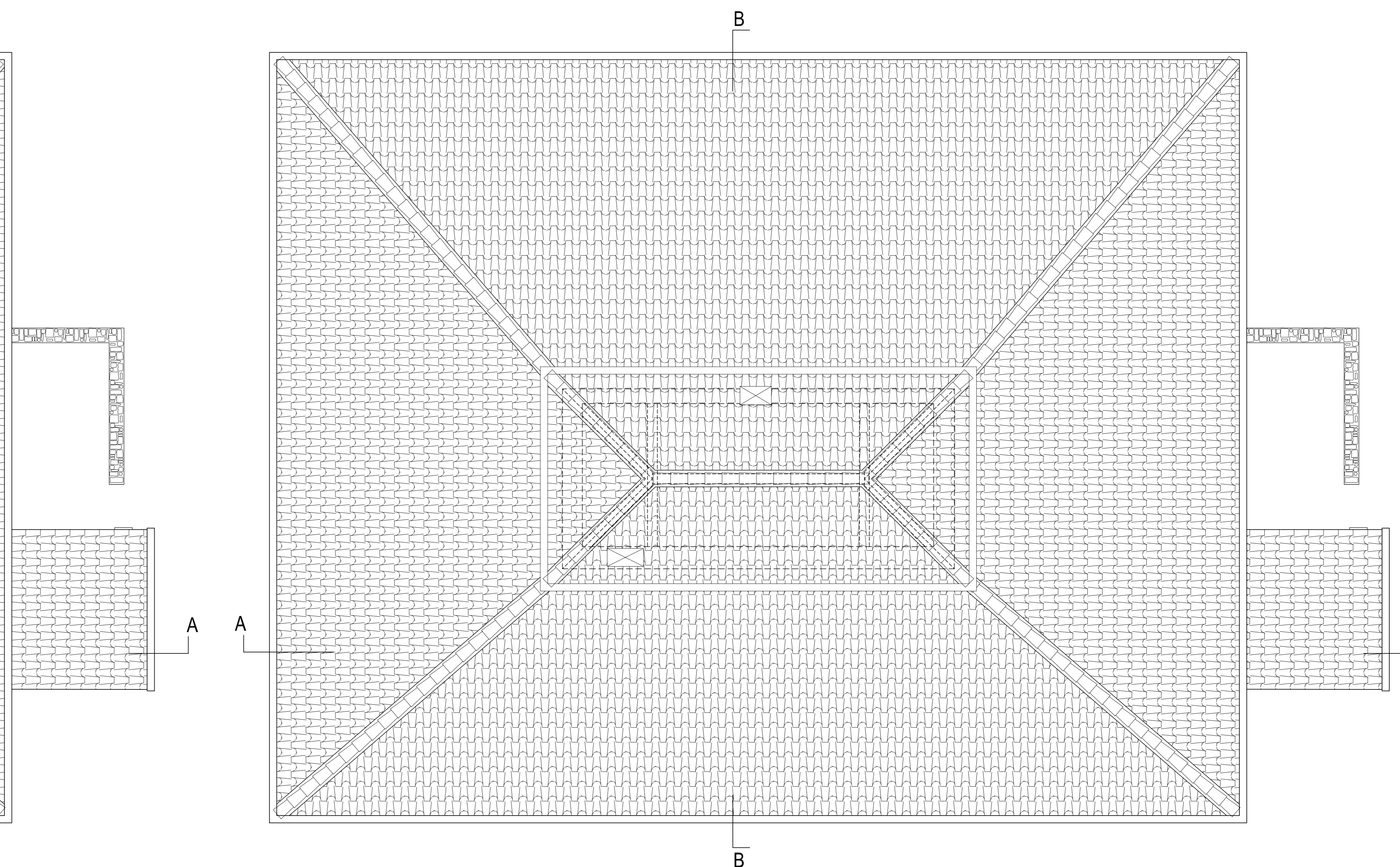
PIANTA COPERTURA DI NUOVA REALIZZAZIONE
