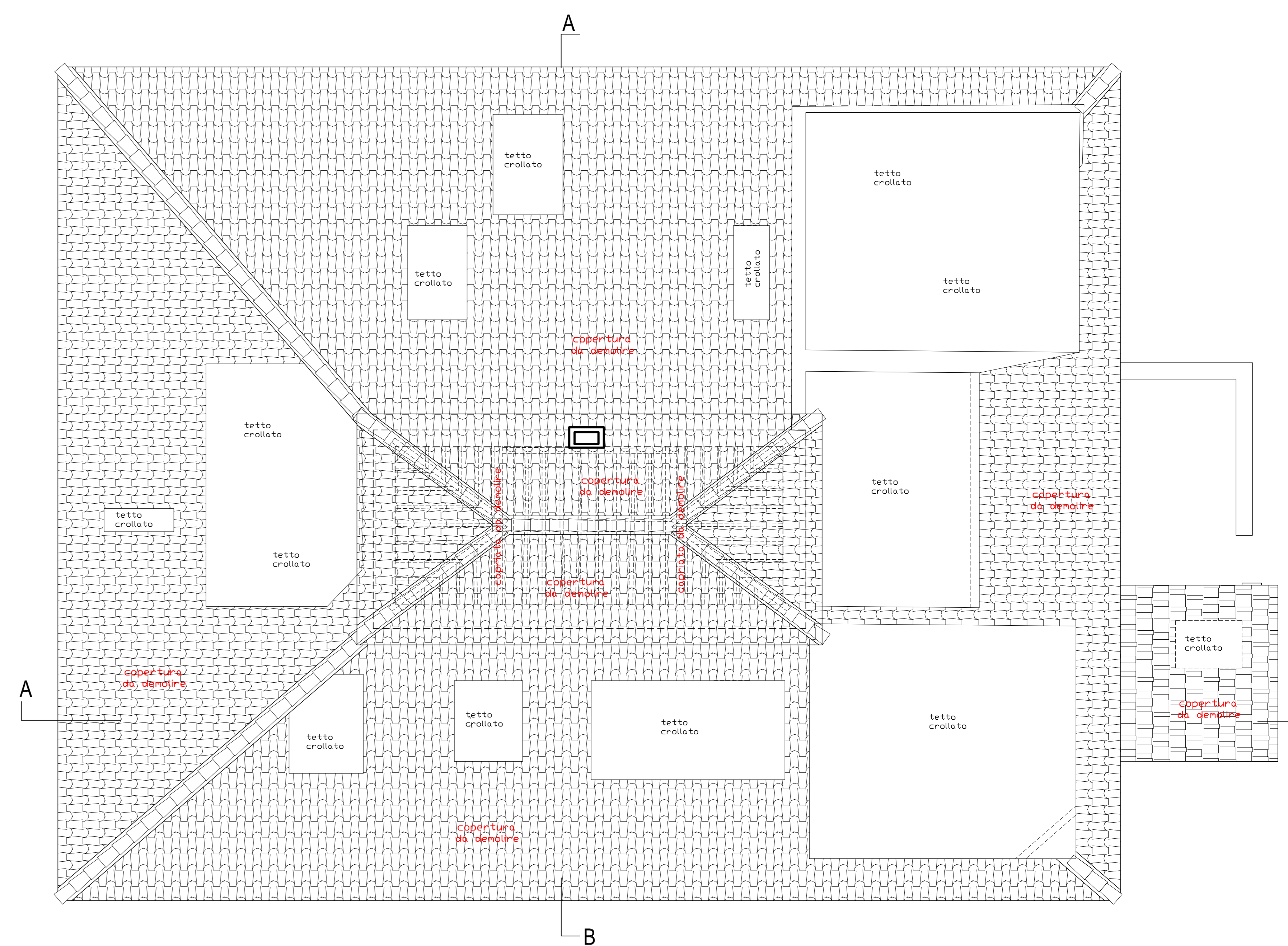
PIANTA COPERTURA
