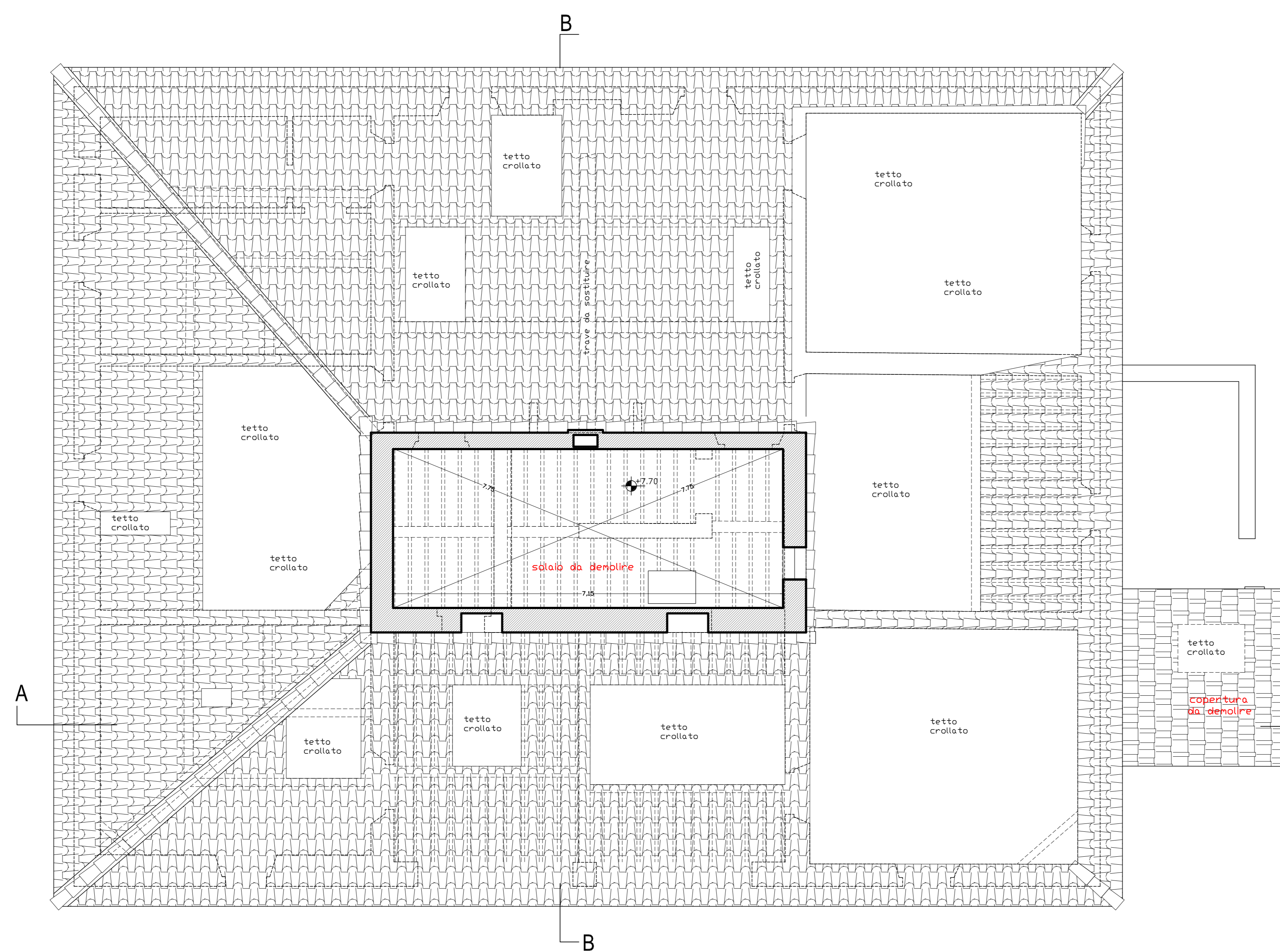
PIANO SECONDO - ALTANA
