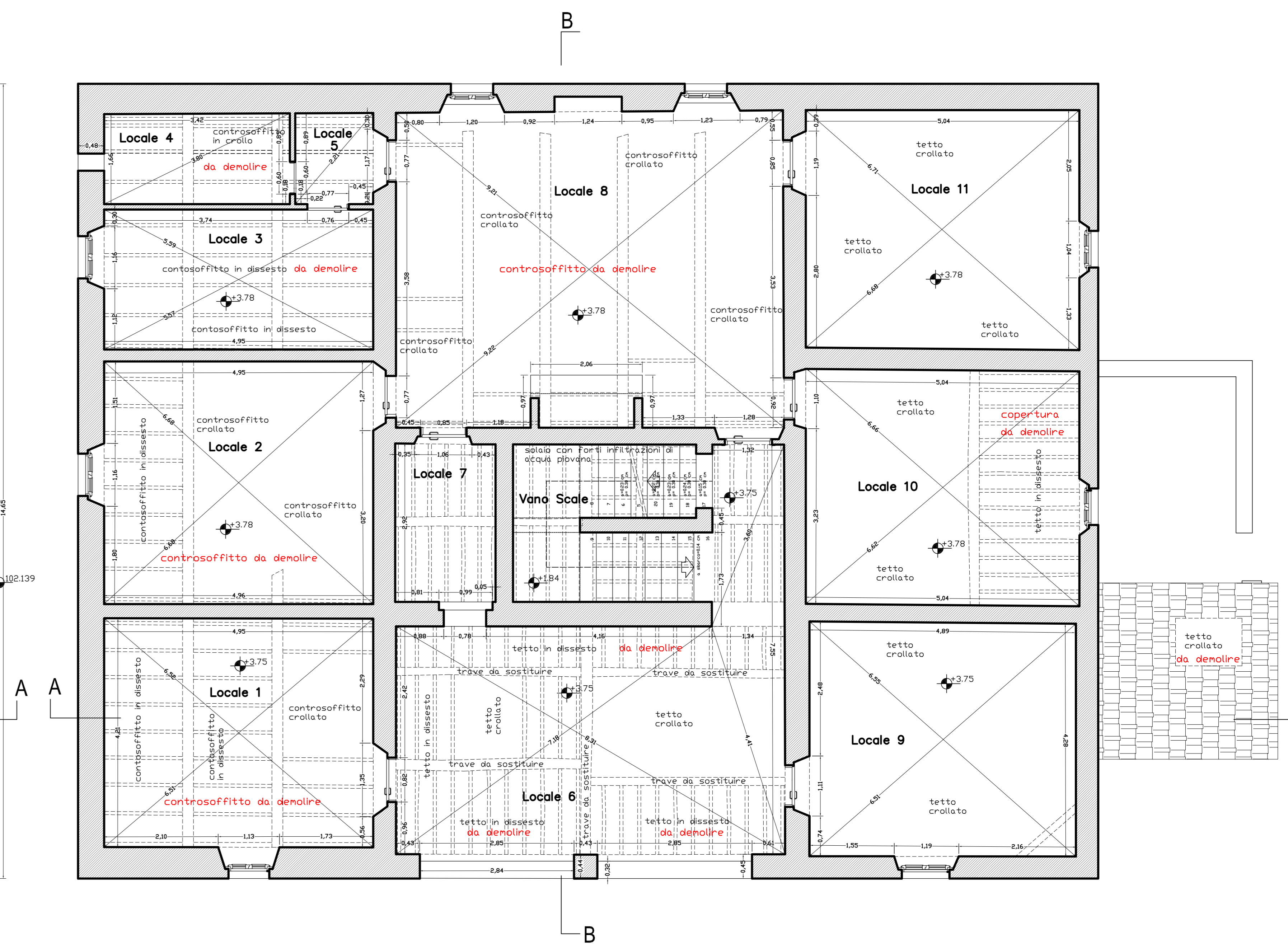
PIANO PRIMO
