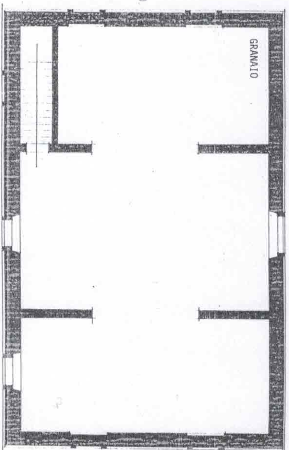
PIANO PRIMO (STATO ATTUALE)
